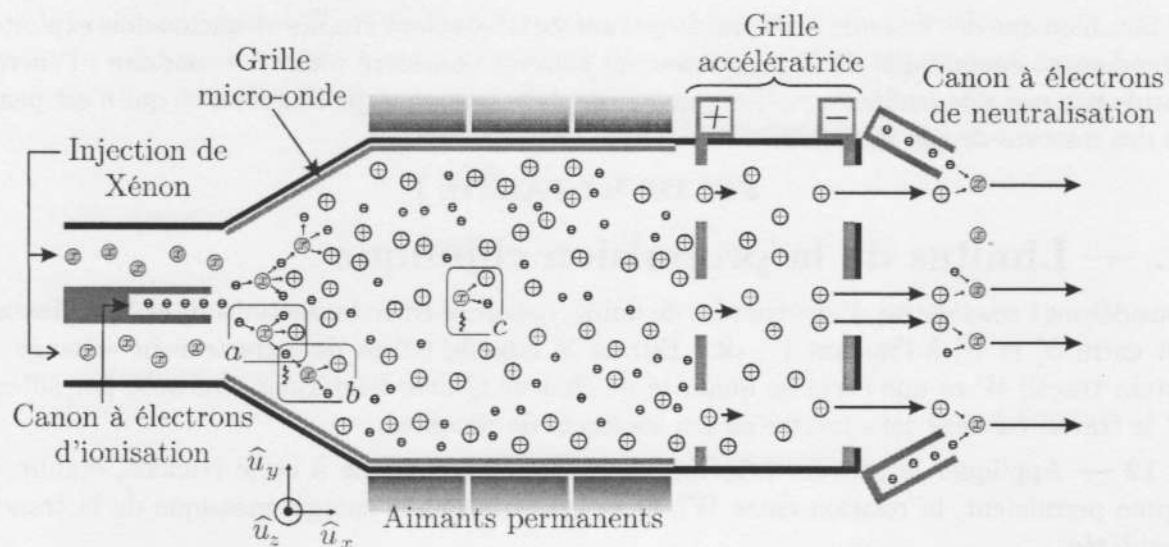
FIGURE 2 — Représentation schématique du moteur ionique : les symboles \odot sont des atomes de Xénon, \oplus des ions \text{Xe}^+ et \bullet des électrons.
