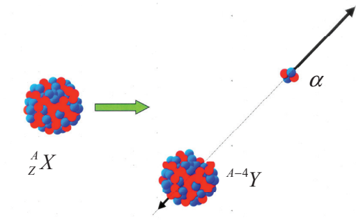
Figure 7 : désintégration \alpha d'un noyau radioactif {}^A_ZX
