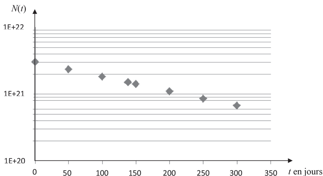
Figure 12 : loi de décroissance radioactive du polonium 210
